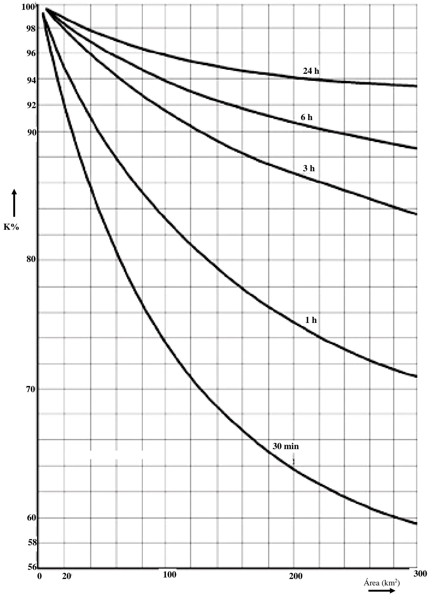
FIGURA 3.7 - COEFICIENTE DE DISTRIBUIÇÃO ESPACIAL DA CHUVA (K)
