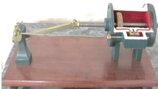
Máquina de pistão a vapor
